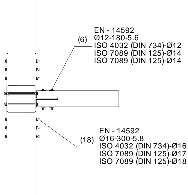
Coupe B-B Échelle 1:20
