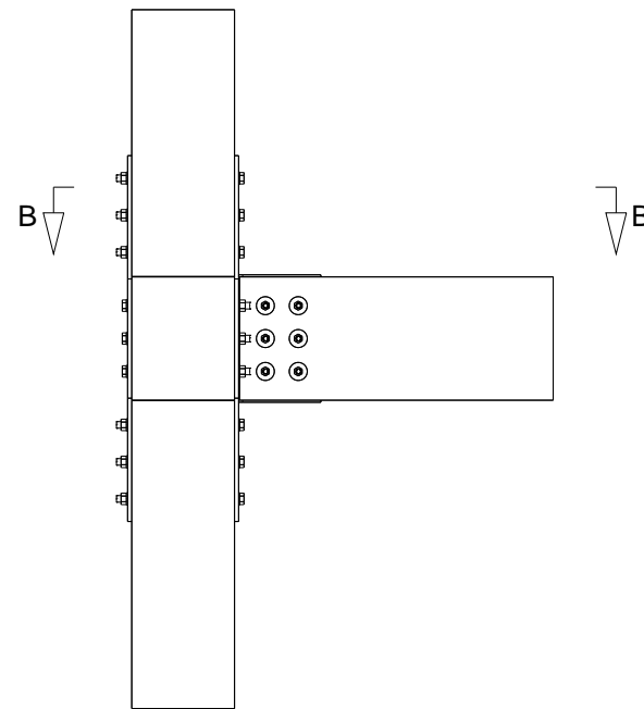
Profil Échelle 1:20
