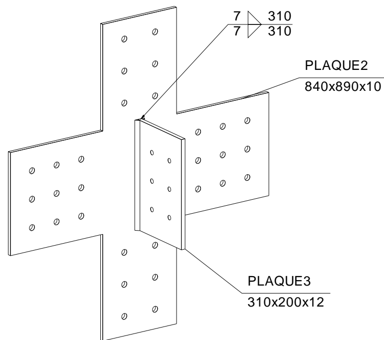
Vue 3D Échelle 1:10
