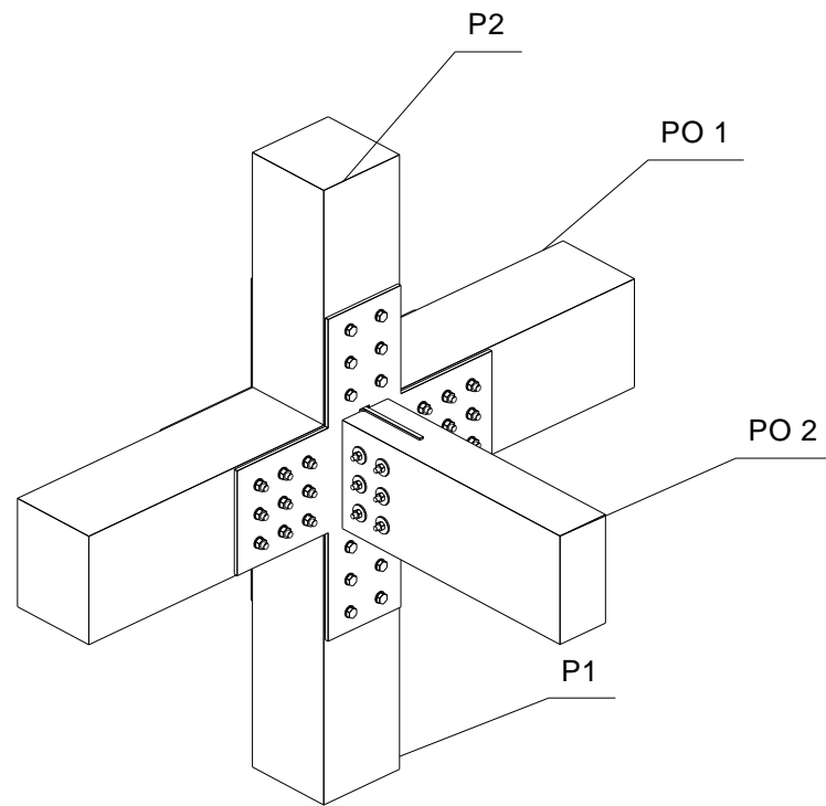
Vue 3D Échelle 1:10
